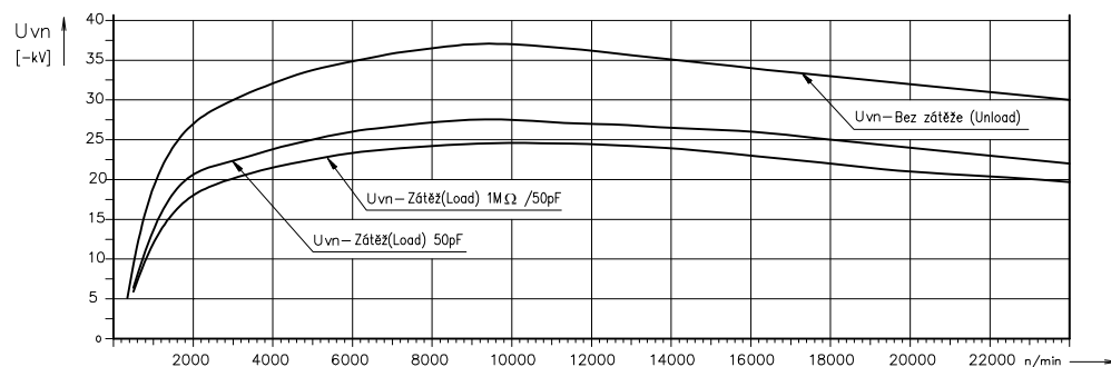
CHARAKTERISTIKA VYSOKÉHO NAPĚTÍ (HIGH VOLTAGE CHARACTERISTIC)
