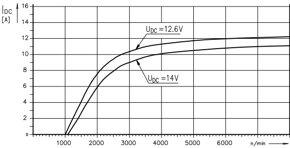
PROVODOVÁ CHARAKTERISTIKA SOUPRAVY
