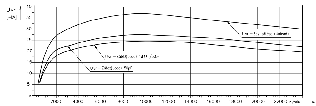
CHARAKTERISTIKA VYSOKÉHO NAPĚTÍ (HIGH VOLTAGE CHARACTERISTIC)
