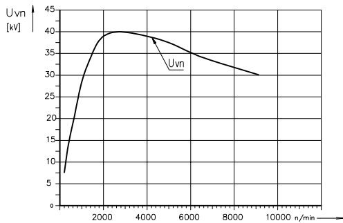
CHARAKTERISTIKA VYSOKÉHO NAPĚTÍ Zátěž 1M Ω /50pF
