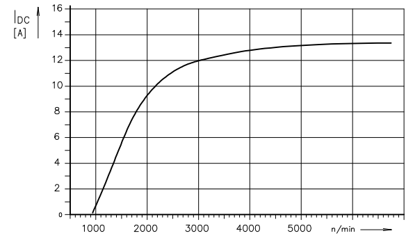
PROUDOVÁ CHARAKTERISTIKA SOUPRAVY
