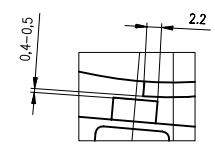
DETAIL POLOHY ROTORU VŮČI SNÍMAČI V OKAMŽIKU PŘESKOKU JISKRY PLATÍ PRO OTAČKY 4000 MIN -1
